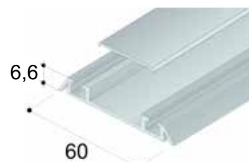
Profil S06NN a krycí profil S06N
